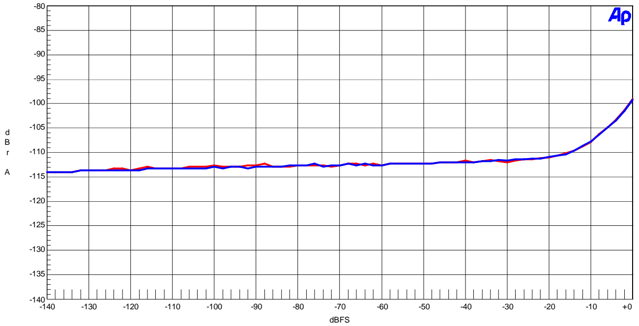
AK4396 THD+N vs Input Level fs=192kHz AVDD=DVDD=5V, 0dBFS input
