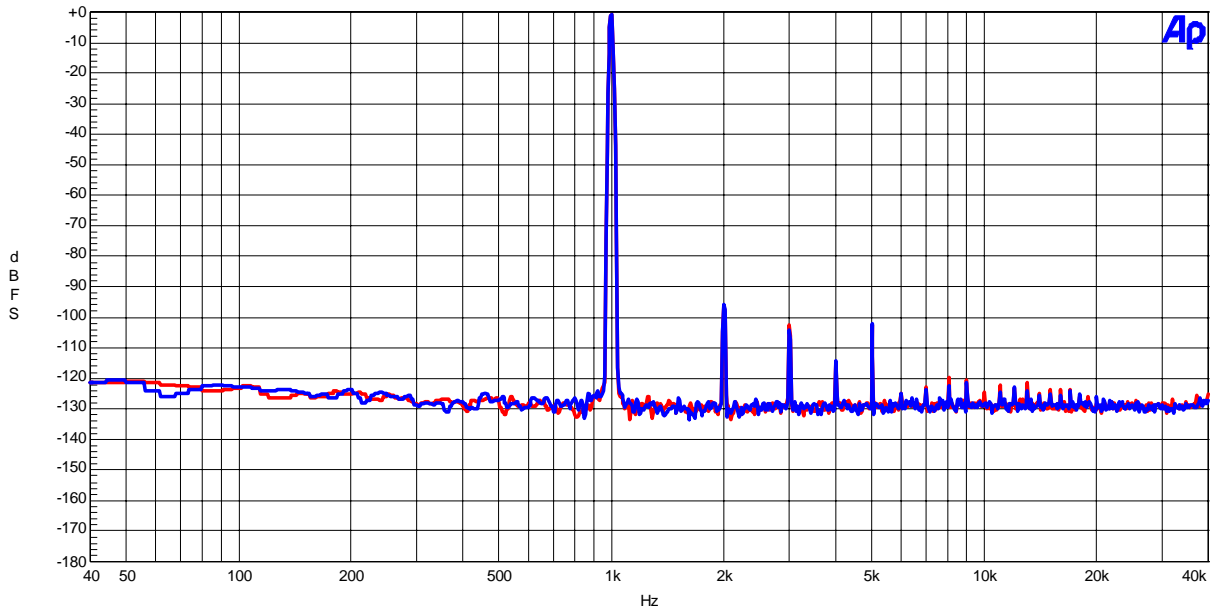
Figure 15 FFT (Input=-0.5dBFS, fin=1kHz)
