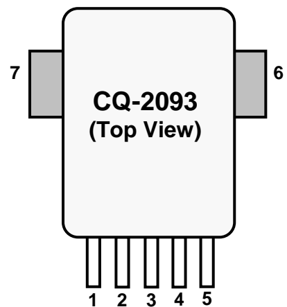
Figure 3. CQ-2093のピン配置図
