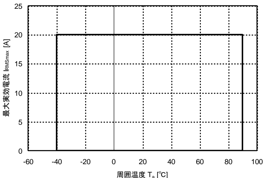
Figure 4. CQ-2093のディレーティングカーブ
