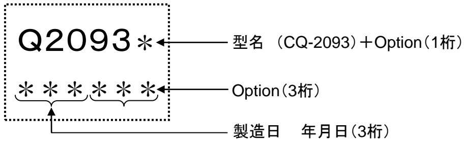
Figure 12. CQ-2093のマーク表示
