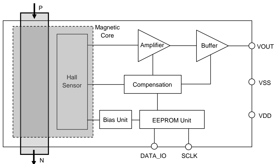
Figure 1. CQ-2093のブロック図
