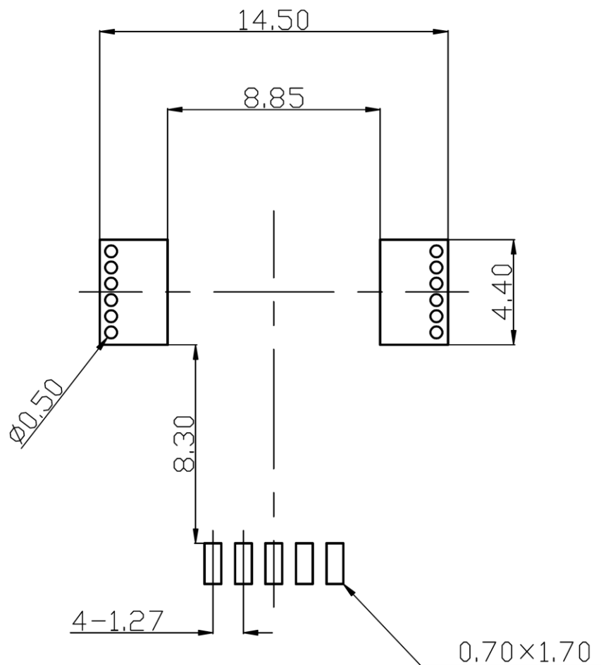
Figure 10. CQ-2093の推奨ランドパターン図
