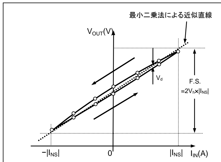
Figure 5. CQ-2093の出力特性
