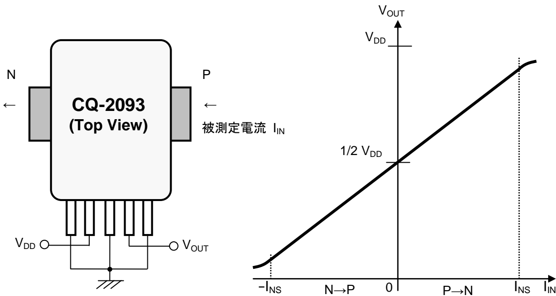
Figure 2. CQ-2093の出力特性
