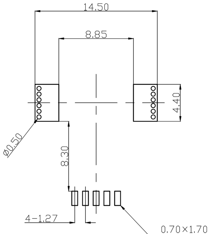
Figure 10. CQ-209Bの推奨ランドパターン図
