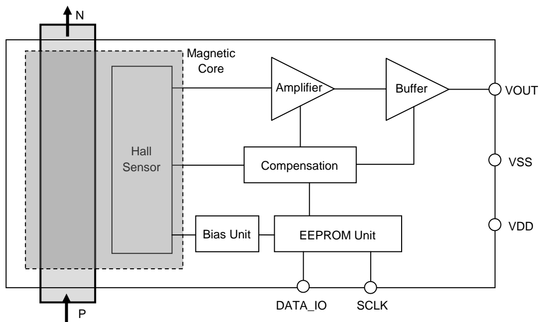
Figure 1. CQ-209Bのブロック図
