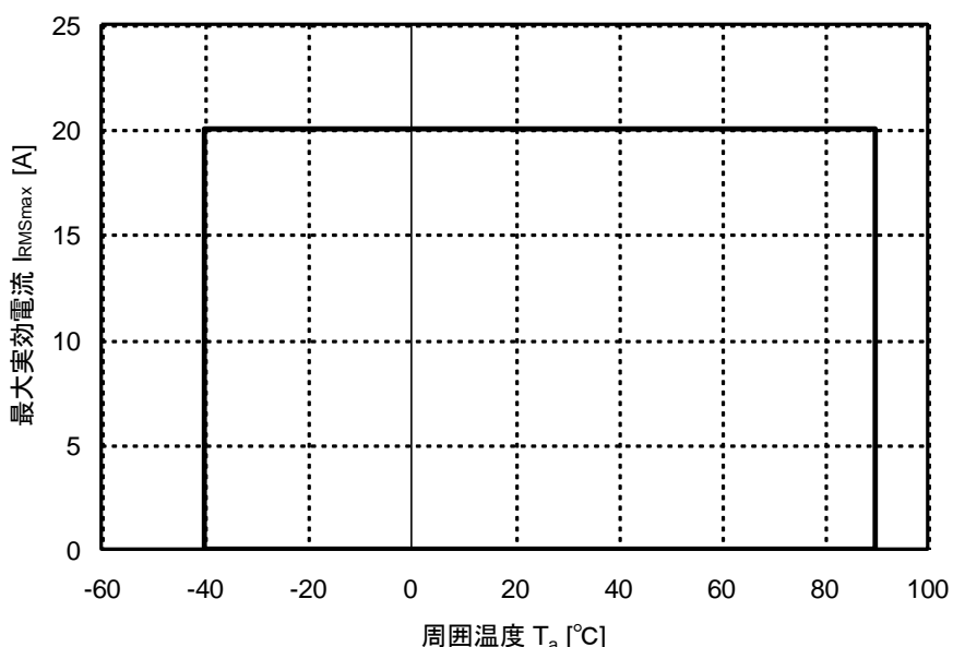
Figure 4. CQ-209Bのディレーティングカーブ
