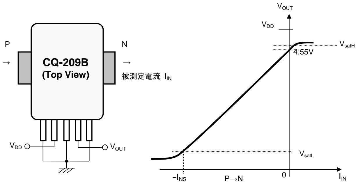
Figure 2. CQ-209Bの出力特性
