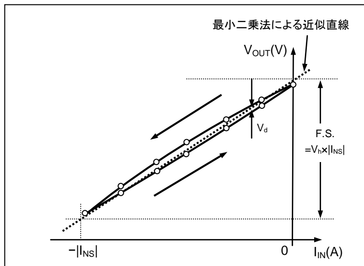
Figure 5. CQ-209Bの出力特性
