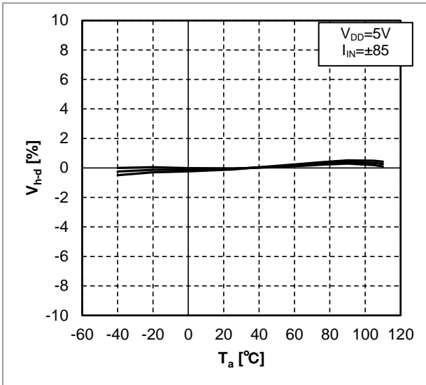
Figure 7. 感度の温度特性 (代表値, n=3)
