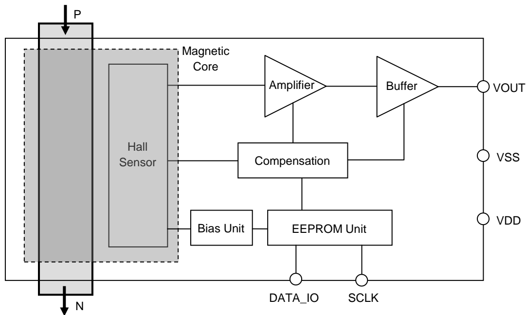
Figure 1. CQ-2335のブロック図
