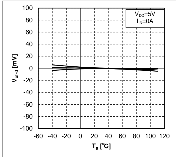
Figure 8. 中点電圧の温度特性(代表値, n=3)
