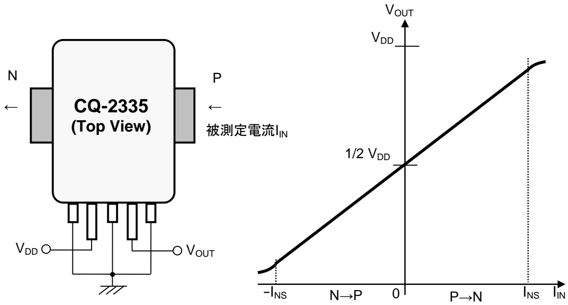
Figure 2. CQ-2335の出力特性
