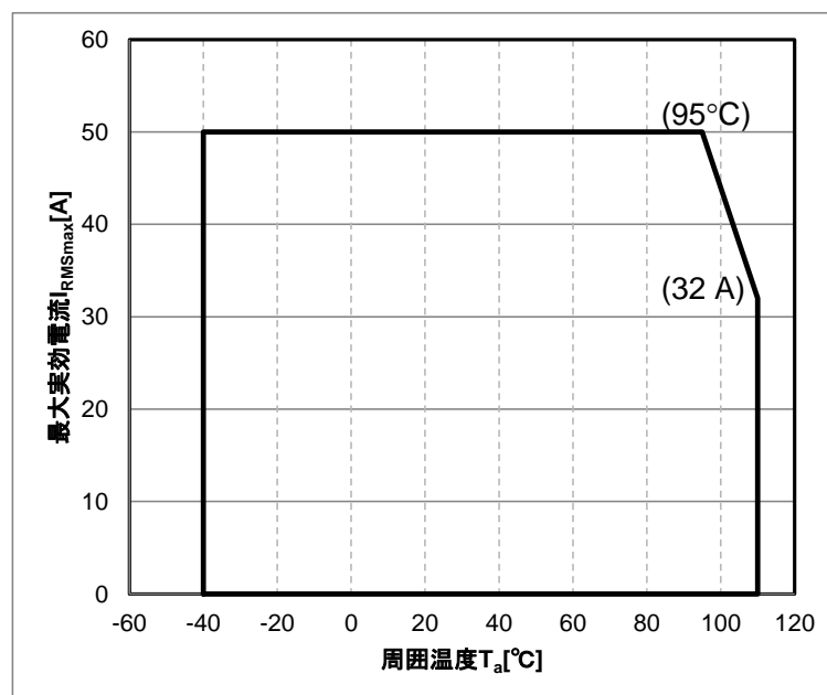
Figure 4. CQ-2335のディレーティングカーブ
