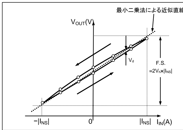
Figure 5. CQ-2335の出力特性
