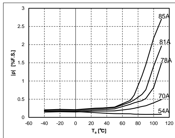
Figure 6. CQ-2335の直線性の温度特性代表値
